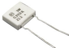
8531 - RES FIO 3 W RADIAL 0R33..... 0,15
