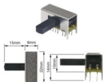
8741 - HORIZ. 16 TERM.ALAV. 15MM MOD.SK43-D03-G15S..... 0.60
