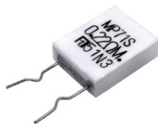
8351 - RES FIO 3 W RADIAL 0R22 ..... 0,15
