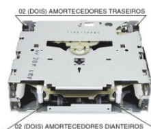
8703 - UNIDADE ÓTICA COM MECANISMO SONY KHM 290AAA..... 40,00
