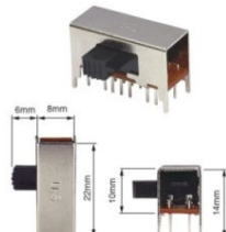
8735 - HORIZ. 16 TERM.ALAV. 6MM MOD.SK42-H02-G6..... 0.60
