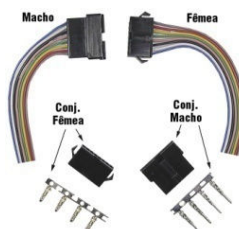
7209 – MINI C/TRAVA, MACHO/ FÊMEA, 8 VIAS P/LINHA AUTOMOTIVA, INFORMÁTICA, ETC. MOD. HX 2522-8..... 0.40 "QTDE. MÍN.10 CONJUNTOS"
