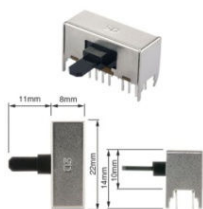
8739 - HORIZ. 16 TERM.ALAV. 11MM MOD.SK43-D01-M12..... 0.60
