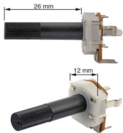
6057 POTENCIÔMETRO 10KB EIXO LONGO (C/ MEIO EIXO ESTRIADO) 3 TERMINAIS 90° SUPORTE TRASEIRO P/MONITORES E USO GERAL ..... 1.60
